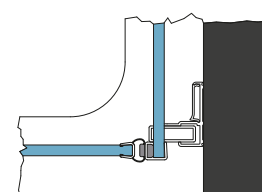
Detal A - widok z góry
