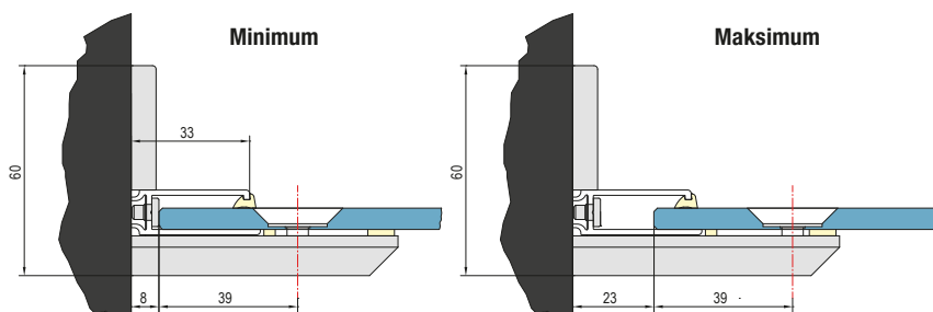
PROFIL PRZYŚCIENNY 50031
