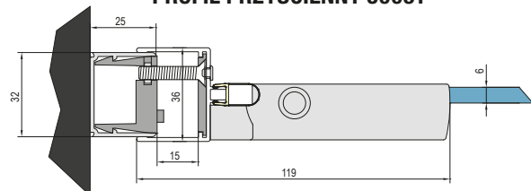
PROFIL PRZYŚCIENNY 50031
