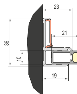
PROFIL ACV2.DU.XX
