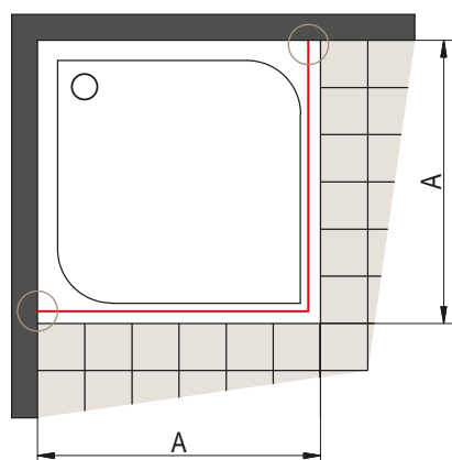
Widok A
