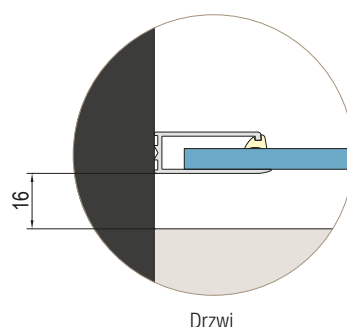
Drzwi
