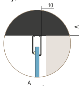
Ścianka boczna 90°
